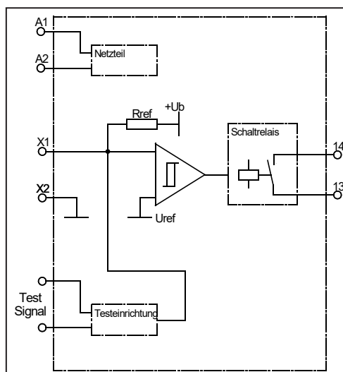
ELMON relay 31-33 Prinzipschaltbild / Simplified diagram
